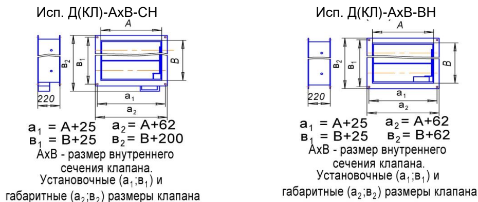
Рис.1. Установочные, габаритные и размеры внутреннего сечения клапана.
