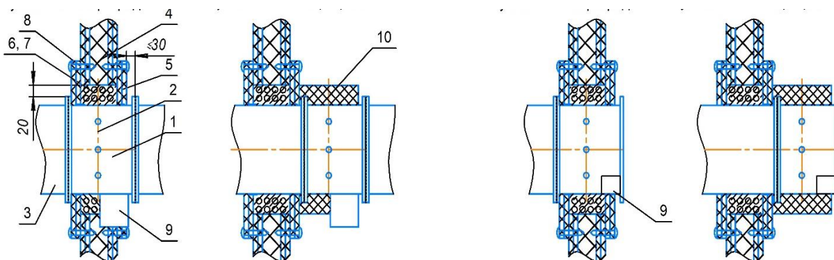
120-Д(КЛ)-СН установка в преграде
